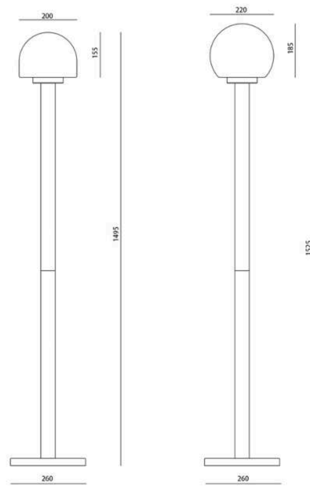
ZT3009-F-A
