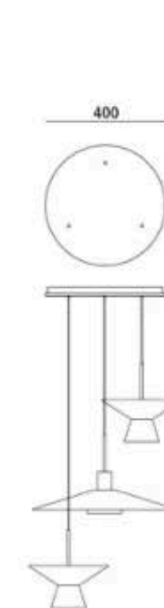
ZT3005-Canopy-D400
