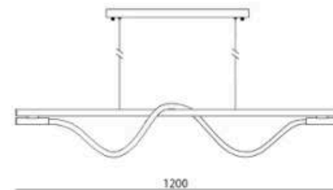
ZT8013-L-12
