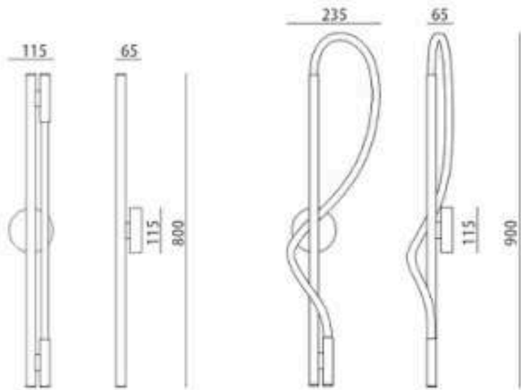
ZT8013-A-M
