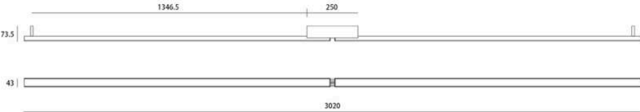
ZT9026-C-3000
