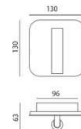
ZT4006-W(B)
